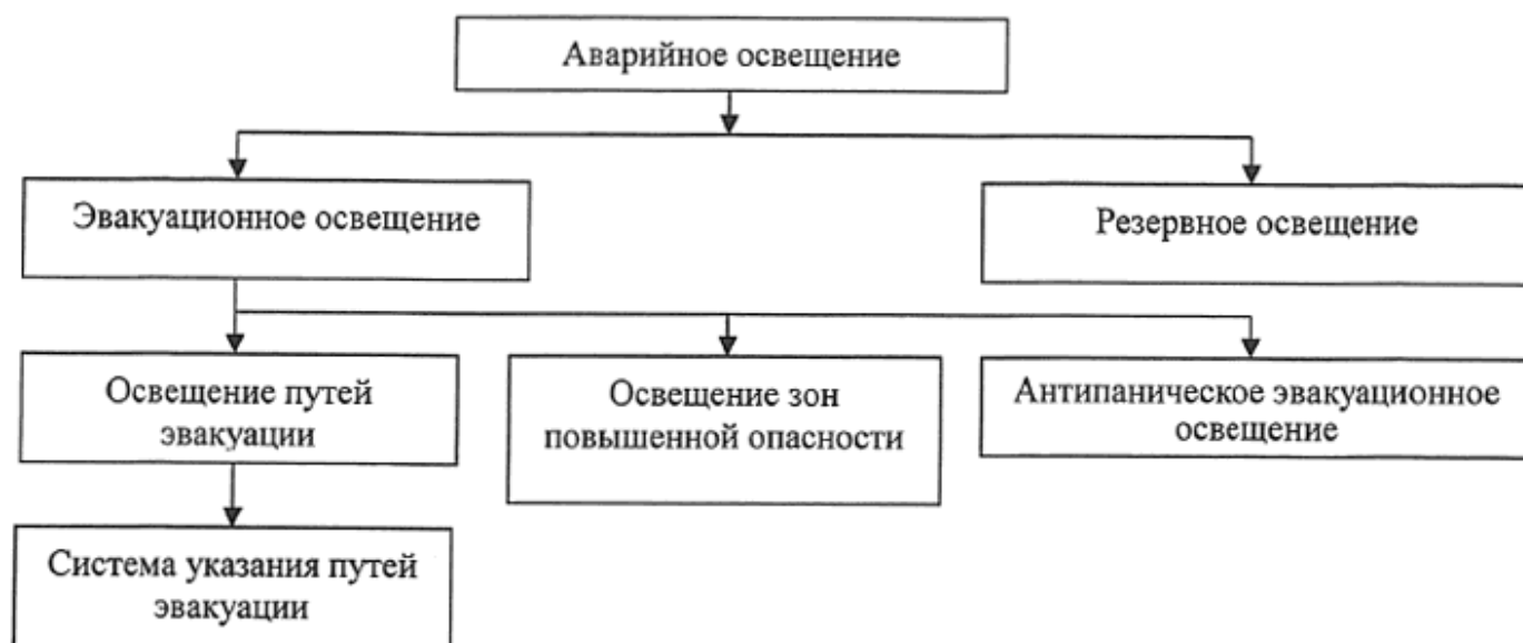
Рисунок 7.1* - Виды аварийного освещения
